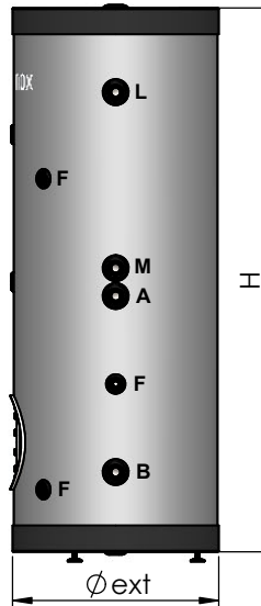
PERFIL DERECHO
