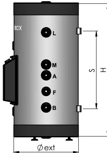
PERFIL DERECHO
